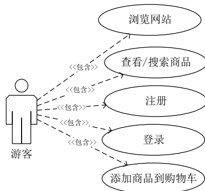
图 3-1 游客用例图
